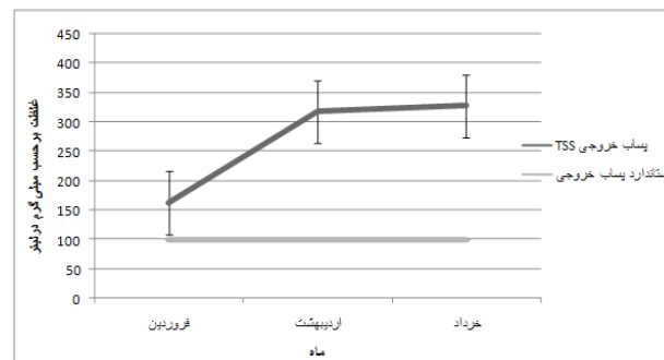
شکل شماره ۳: میانگین تغییرات TSS خروجی تصفیه خانه در سه ماهه ی اول سال و مقایسه آن با استاندارد
