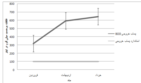
شکل شماره ۱: میانگین تغییرات BOD خروجی تصفیه خانه در سه ماهه ی اول سال و مقایسه آن با استاندارد
